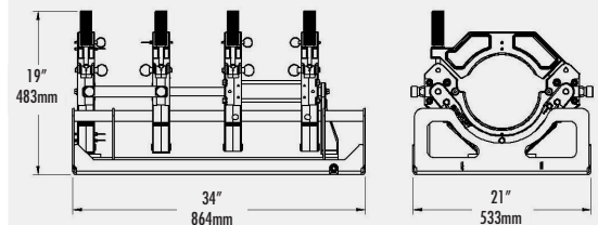
DYNAMC 250 EP 4-JAW
