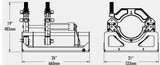
DYNAMC 250 EP 2-JAW
